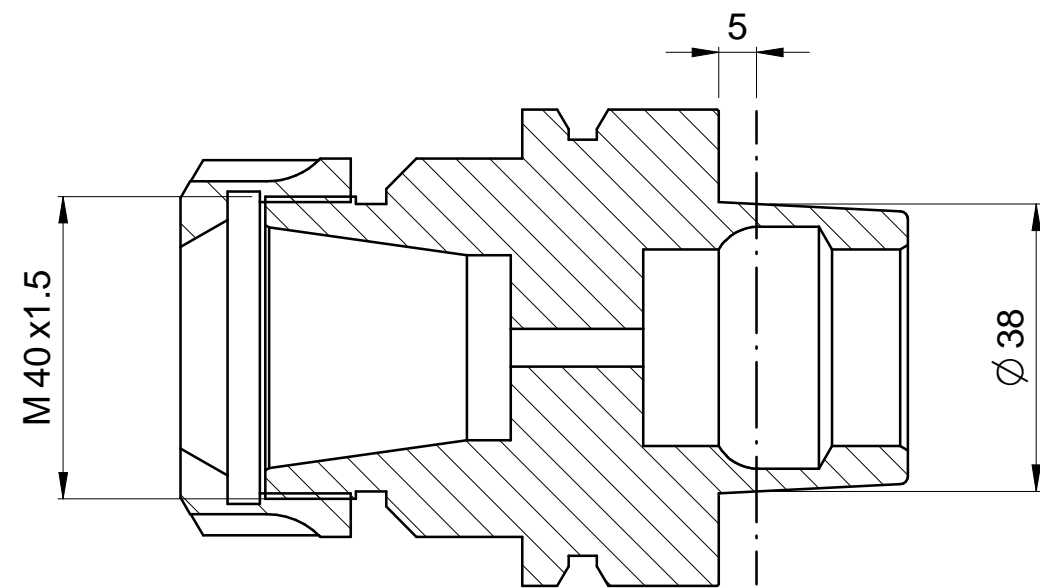
SEZIONE A-A
